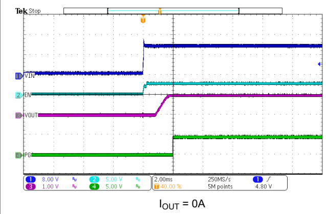
图 7-13. VIN Start-Up
