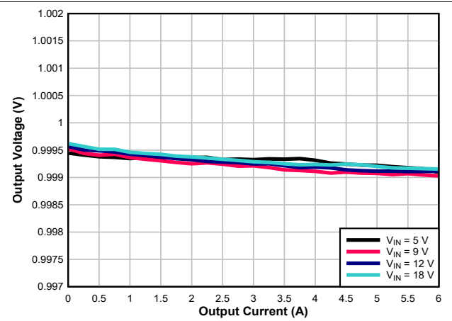
图 7-5. Load Regulation
