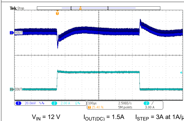
图 7-8. Load Transient
