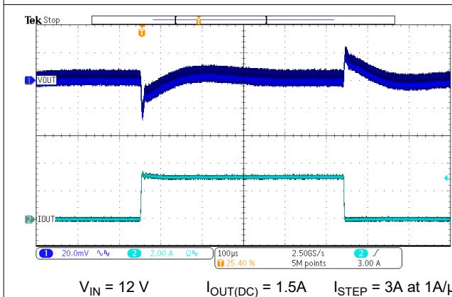
图 7-8. Load Transient
