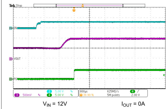
图 7-12. EN Start-Up - 0.5V Prebias
