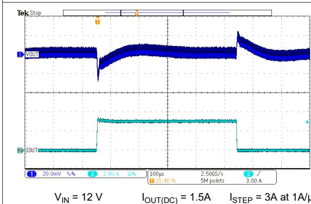
图 7-8. Load Transient
