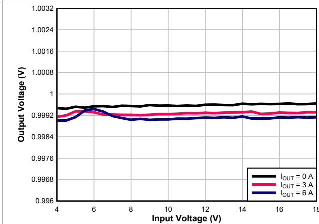
图 7-6. Line Regulation
