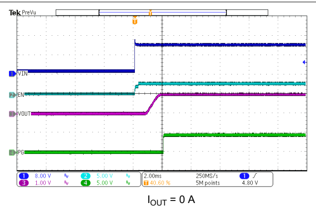
图 7-13. VIN Start-Up
