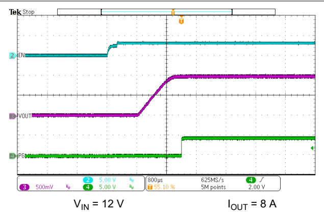
图 7-11. EN Start-Up - With Load
