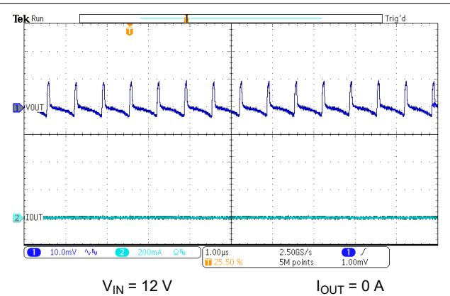
图 7-15. Output Ripple - No Load
