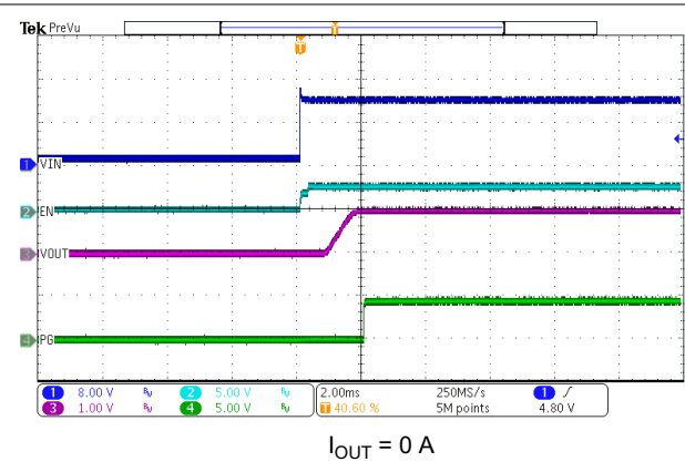
图 7-13. VIN Start-Up
