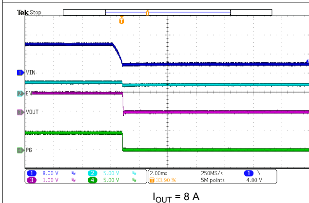
图 7-14. VIN Shutdown
