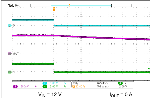
图 7-10. EN Shutdown No Load
