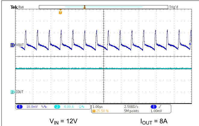
图 7-16. Output Ripple – 8A Load
