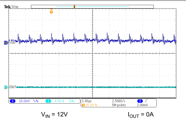
图 7-17. Input Ripple – No Load
