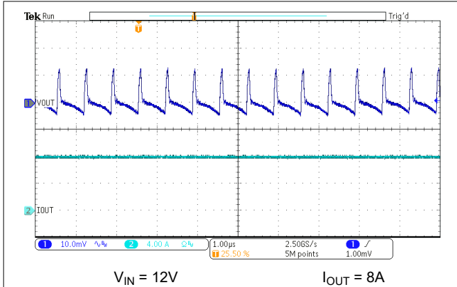
图 7-16. Output Ripple – 8A Load
