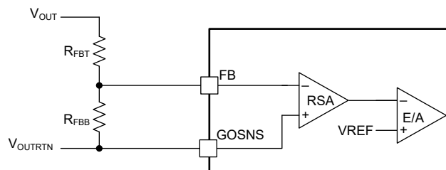
图 7-5. FB 电阻分压器
