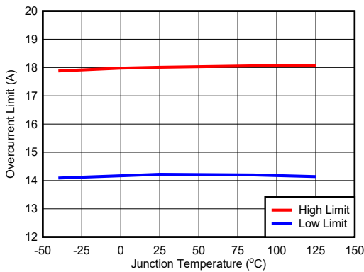
图 6-3. 过流限值
