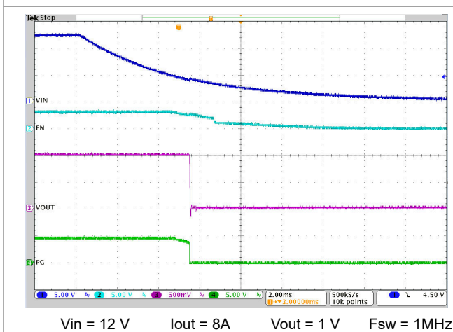
图 8-14. VIN 关断
