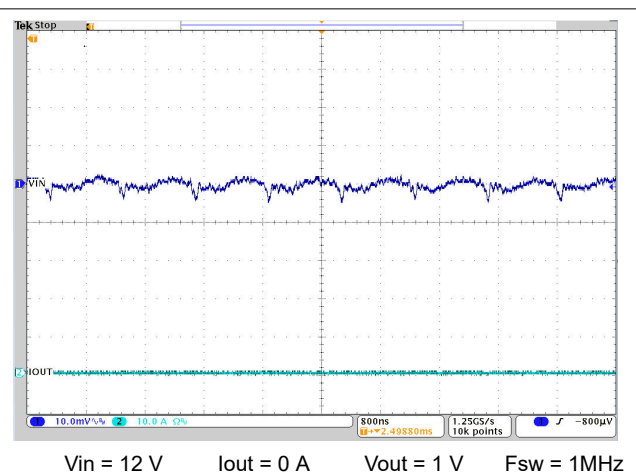
图 8-15. 输入纹波 - 空载
