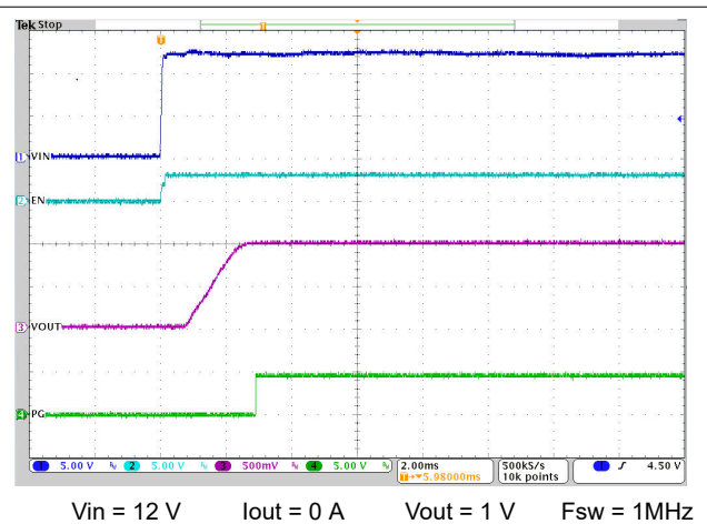
图 8-13. VIN 启动
