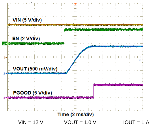
图 9. EN Start-up Waveforms
