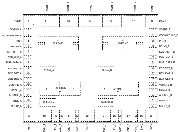
图 4-1. 59-Pin QFM-MOW Package (Top View)
