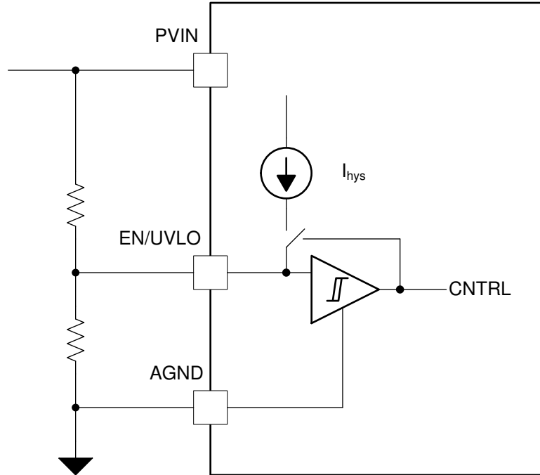
图 6-5. TPSM8D6C24 UVLO Voltage Divider
