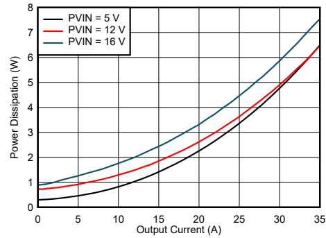
图 7-4. Power Dissipation
