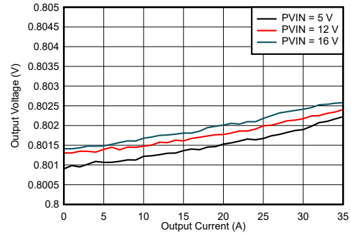
图 7-2. Load Regulation
