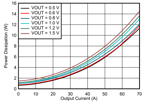
图 5-8. TPSM8D6C24 Power Dissipation vs Output Current
