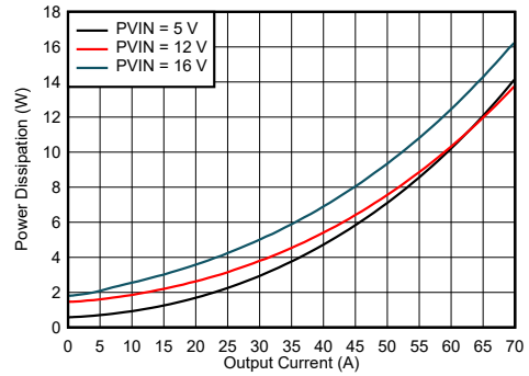
图 7-13. Power Dissipation
