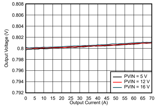
图 7-11. Load Regulation
