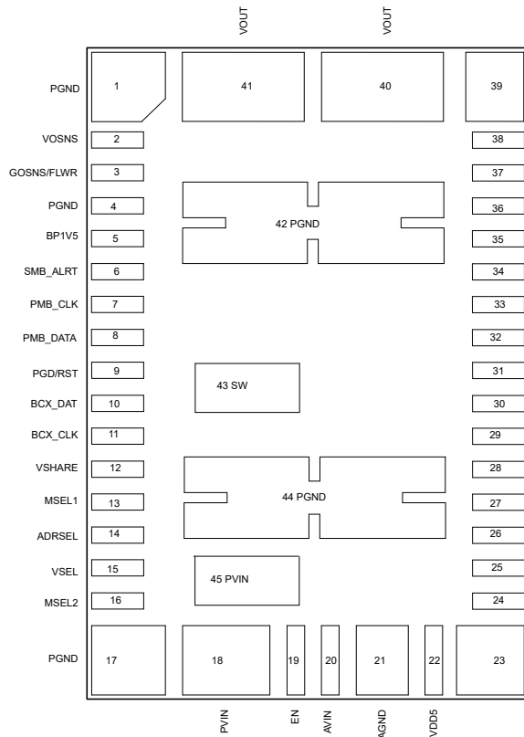
图 4-1. 45-Pin QFM-MOY Package (Top View)
