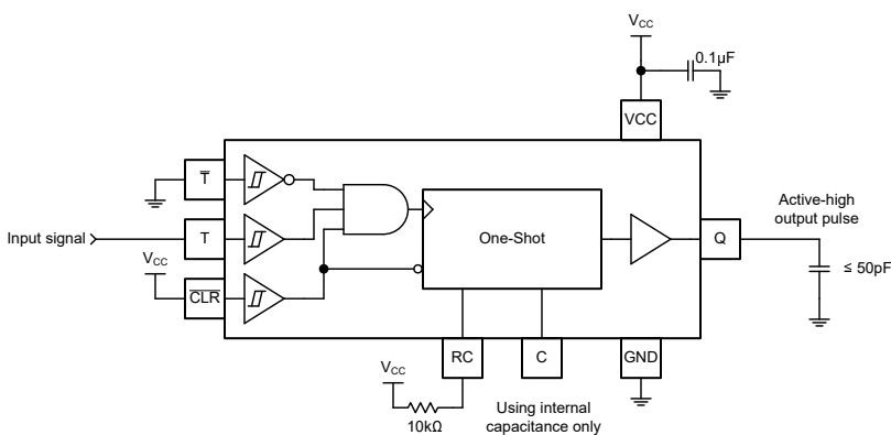
图 8-3. 使用 TPUL1G113 进行上升沿检测
