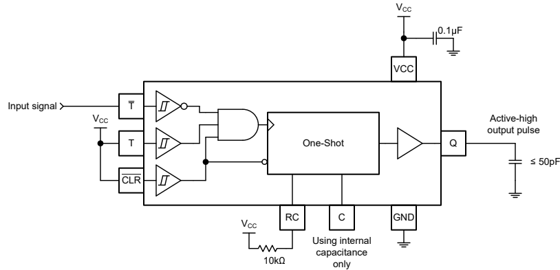
图 8-4. 使用 TPUL1G113 进行下降沿检测
