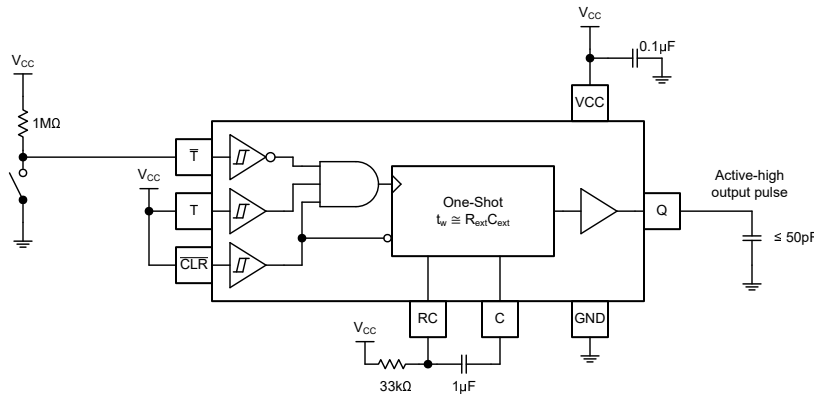
图 8-5. 使用 TPUL1G113 对开关进行去抖
