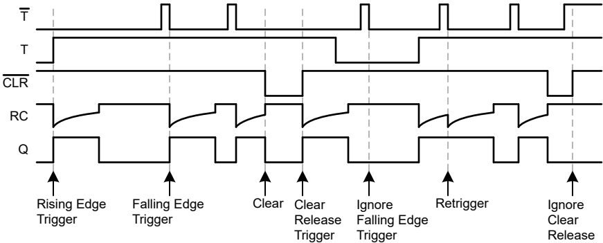
图 5-1. 时序图
