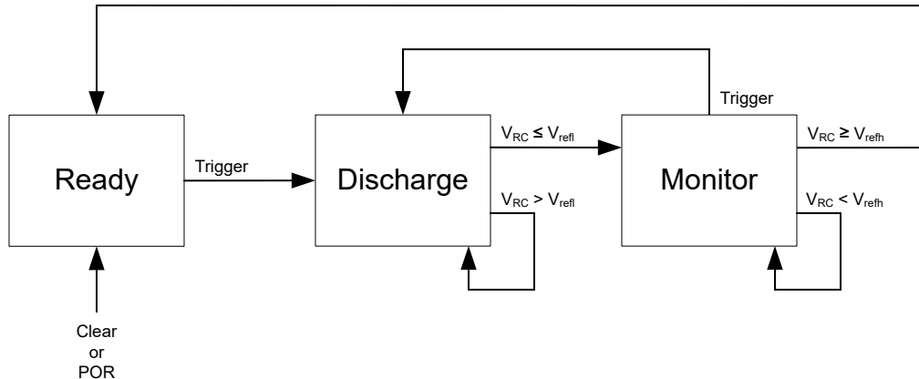
图 7-3. 状态机图
