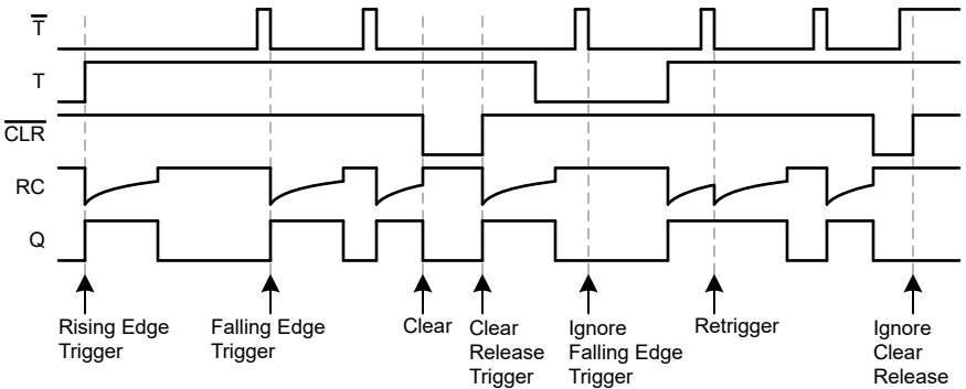
图 5-1. 时序图
