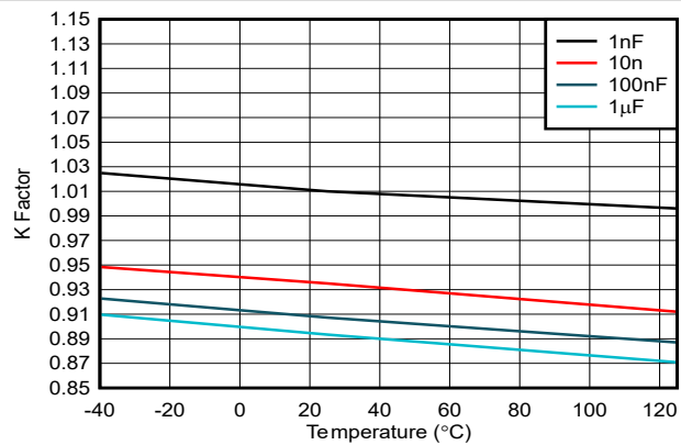
图 5-6. K 系数与温度间的关系, R_{ext} = 10k \Omega
