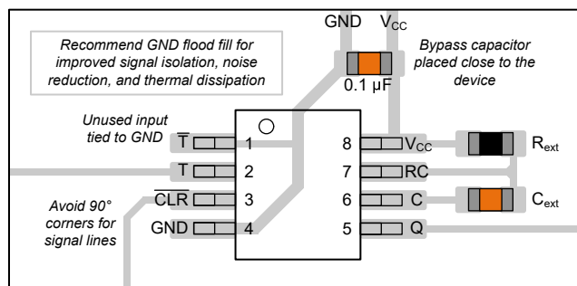
图 8-3. 布局示例
