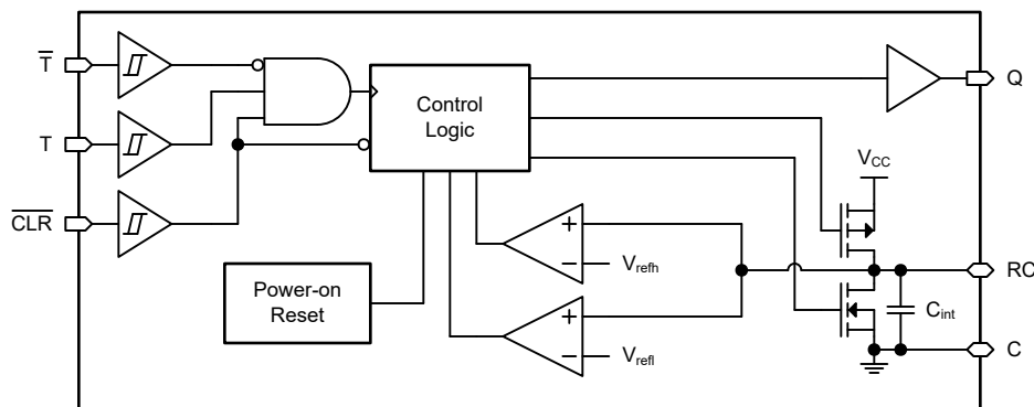
图 7-4. 功能方框图
