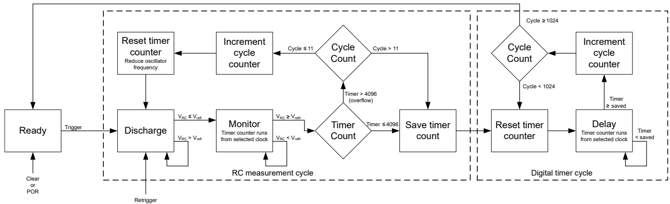
图 7-3. 状态机图
