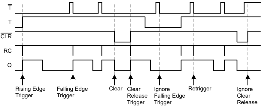
图 5-1. 时序图
