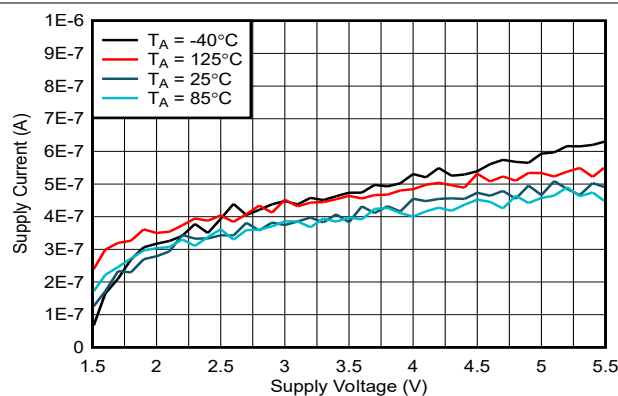
图 5-2. 电源电流与电源电压间的关系
