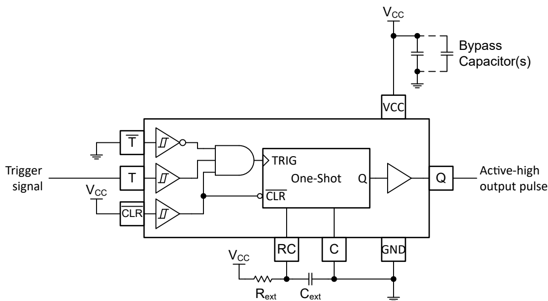
图 8-1. 使用 TPUL1G313-Q1 生成脉冲
