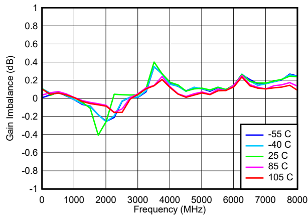
图 6-25. Gain Imbalance
