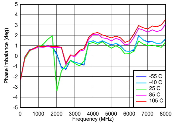
图 6-26. Phase Imbalance
