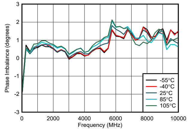
图 5-32. 相位不平衡
