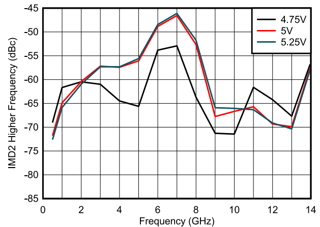
图 5-20. 整个 V_{DD} 范围内的 IMD2 更高
