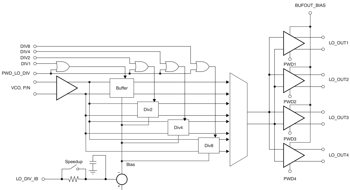
Figure 68. LO Divider
