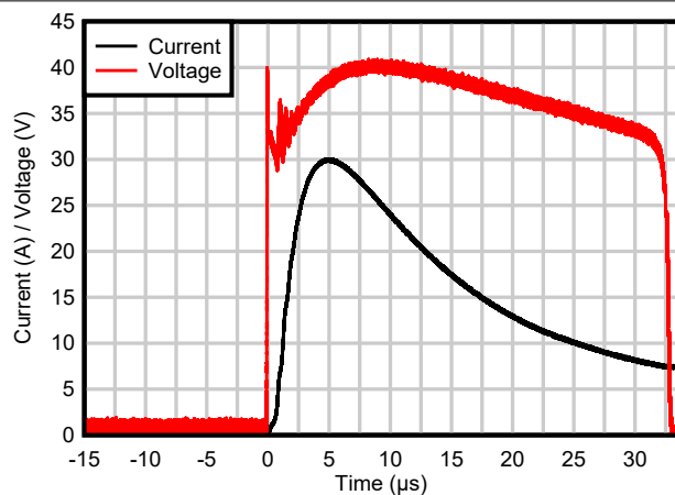
图 6-1. 8/20 \mu s 浪涌响应
