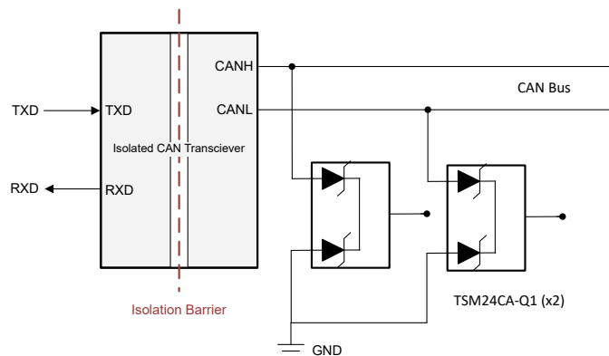
电动汽车充电 CAN 总线应用
