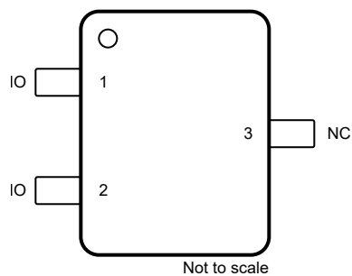
图 5-1. DBZ 封装，3 引脚 SOT-23 ( 顶视图 )
