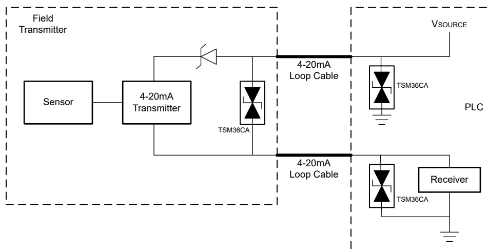
图 6-1. 典型应用图
