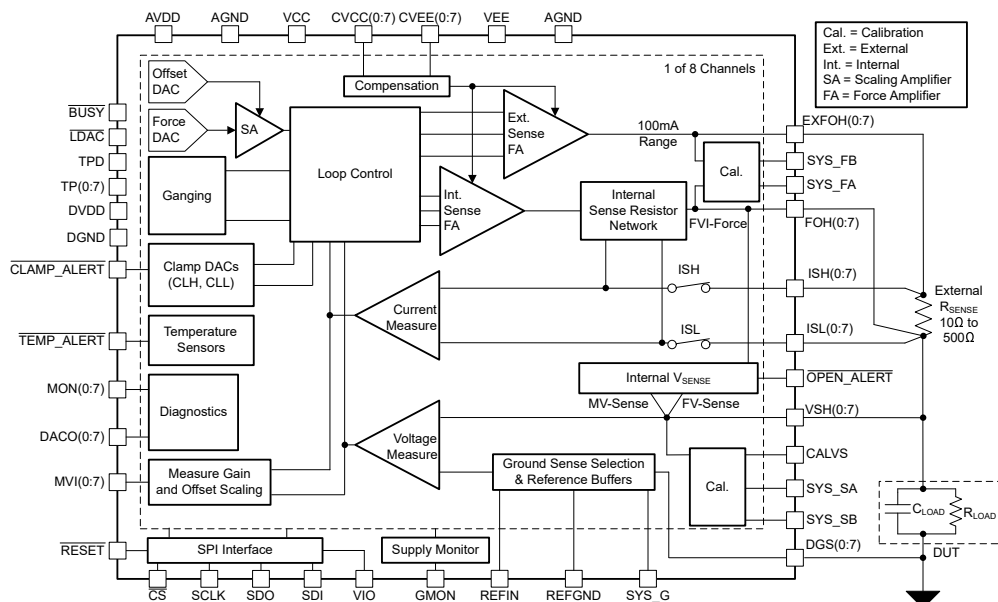
方框图
