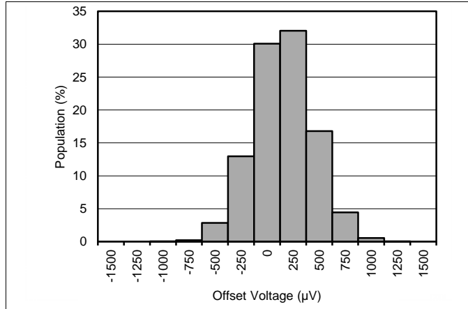
图 1. 失调电压产生分布
