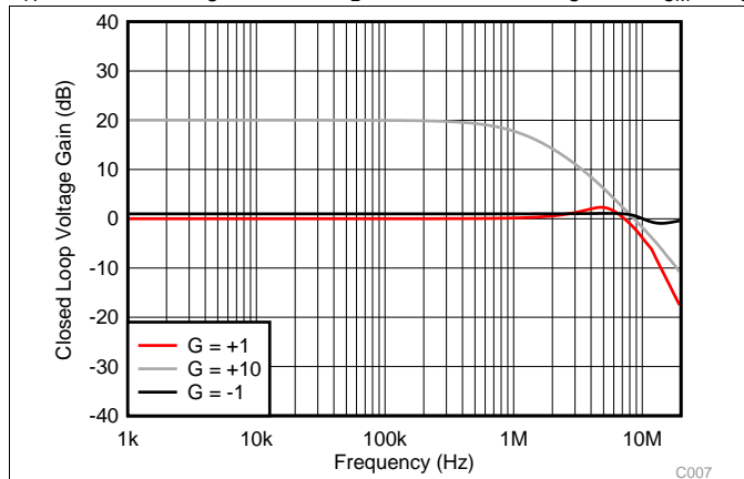
图 7. 闭环增益与频率间的关系
