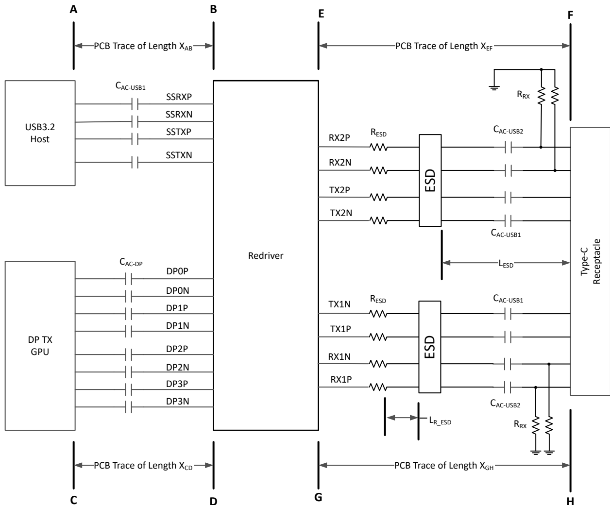
图 8-1. TUSB5461-Q1 在主机应用中
