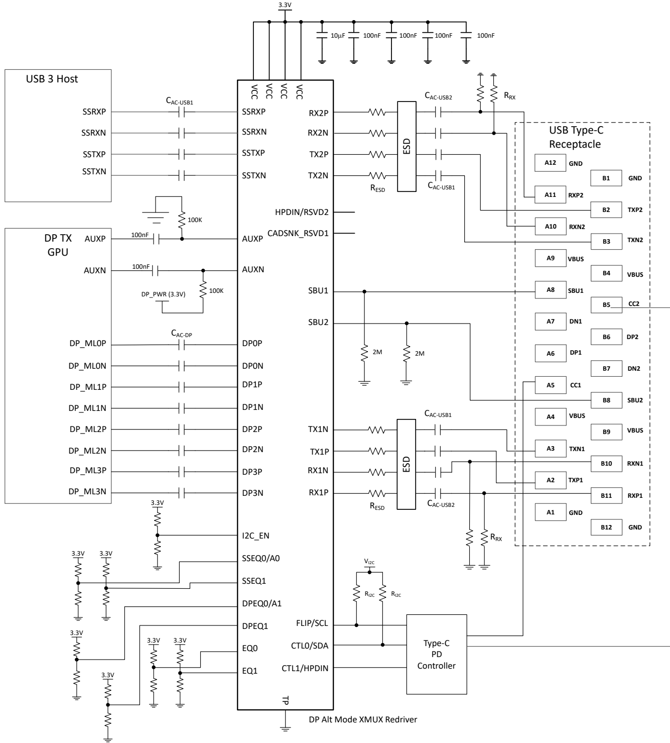
图 8-2. 应用电路
