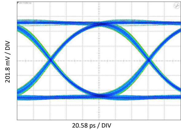
图 5-12. 8.1Gbps 下具有 12 英寸输入 PCB 布线的 DisplayPort HBR3 眼图性能
