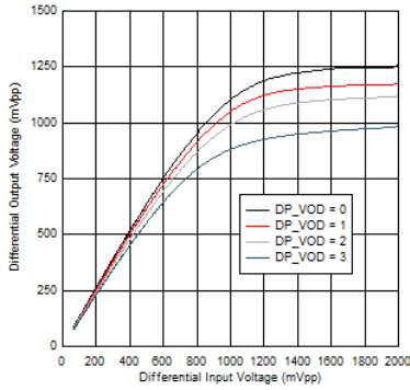
图 5-13. 100MHz 下的 DP VOD 线性设置
