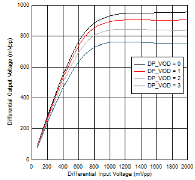
图 5-14. 5GHz 下的 DP VOD 线性设置
