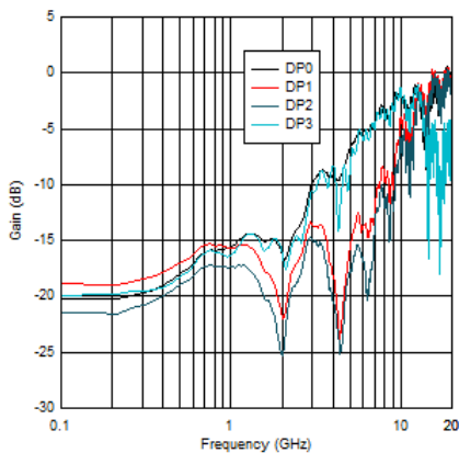
图 5-11. DisplayPort 输出回波损耗性能
