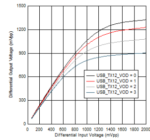
图 5-16. 100MHz 下的 USB TX1 VOD 线性设置
