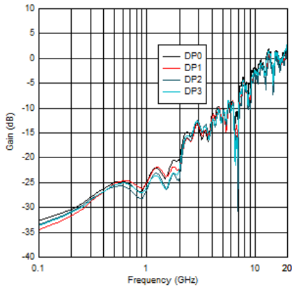
图 5-9. DisplayPort 输入回波损耗性能
