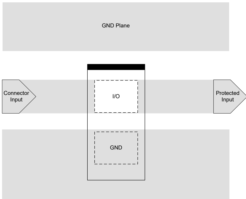
图 6-1. TVS2210 布局
