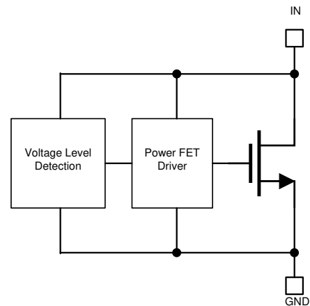
功能方框图
