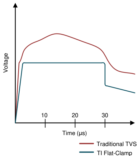
对 8 \mu s 至 20 \mu s 浪涌事件的电压钳位响应
