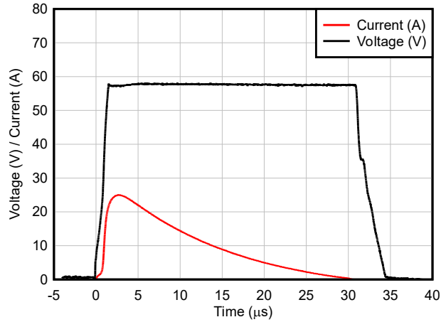
图 6-1. 电流为 25A 时，浪涌响应为 8/20μs
