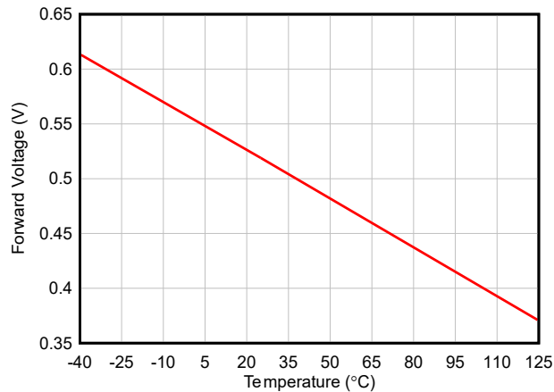
图 6-3. 正向电压与温度间的关系
