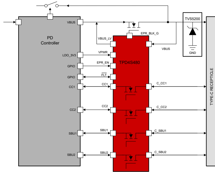
图 8-1. TVS5200 应用原理图
