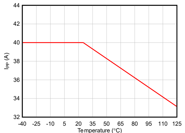
图 6-6. 最大浪涌电流 (8/20 \mu s) 与温度间的关系
