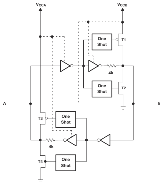
图 7-1. TXB0104W I/O 单元架构
