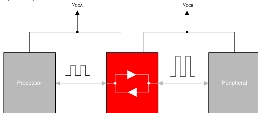
TXB0104W 典型应用方框图
