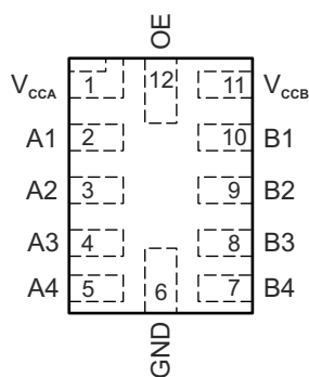
图 4-1. RUT 封装 (顶视图)
