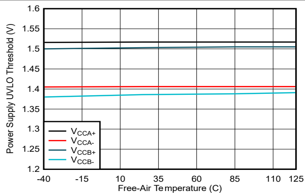
图 5-8. 电源欠压阈值与自然通风条件下的温度间的关系
