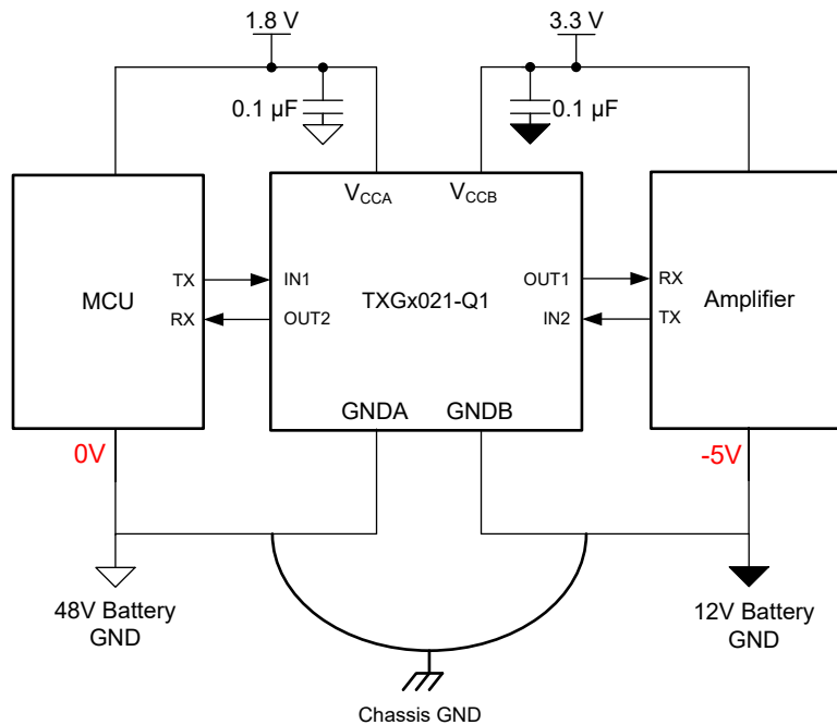
图 8-1. 汽车中的 TXG4021-Q1
