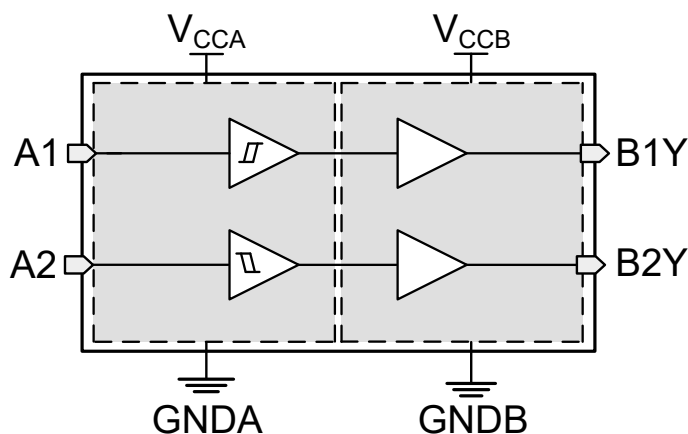
图 7-2. TXG4020-Q1 功能方框图
