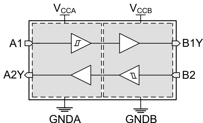
图 7-1. TXG4021-Q1 功能方框图
