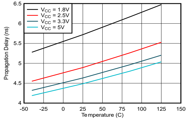
图 5-7. 传播延迟 T_{PHL} 与温度间的关系
