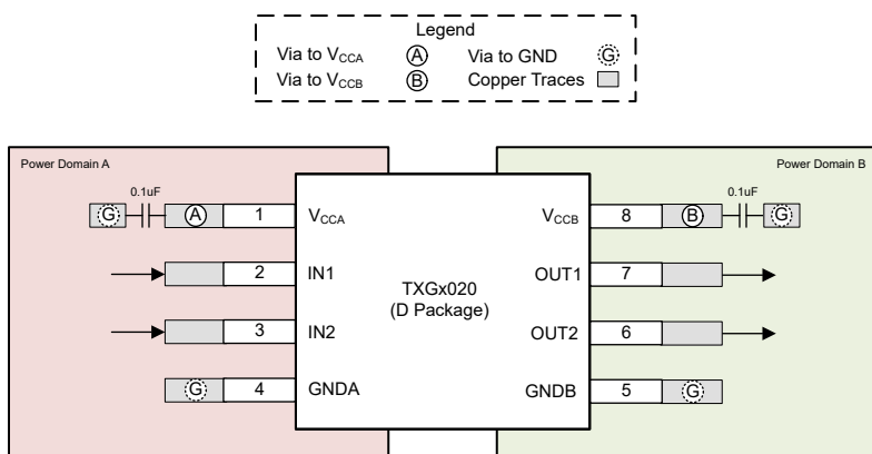
图 8-3. D 布局示例
