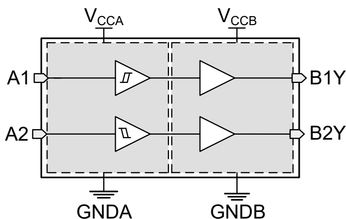
图 7-2. TXG4020 功能方框图
