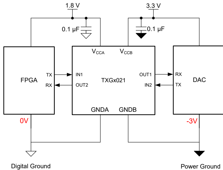
图 8-1. 测试和测量中的 TXG4021
