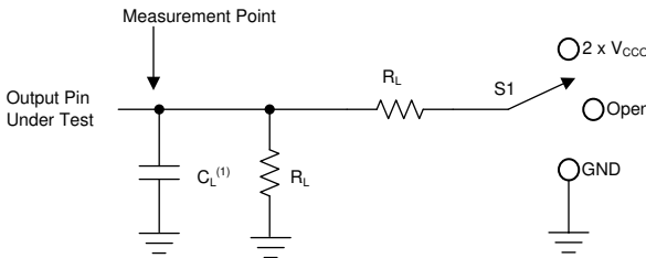
图 6-1. 负载电路
