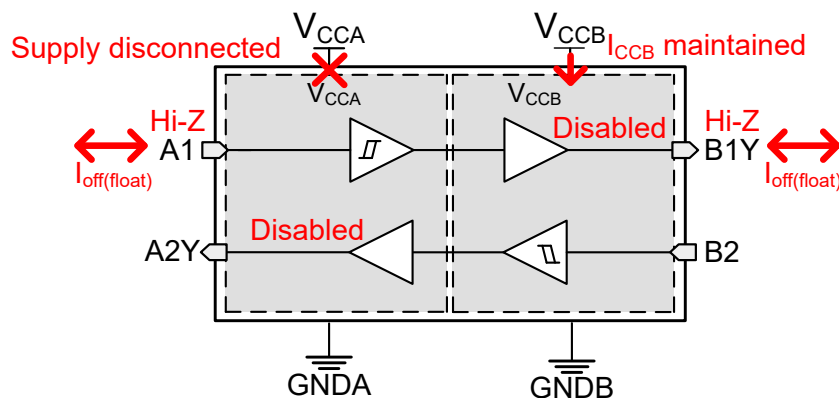
图 7-3. V_{CC} 断开特性
