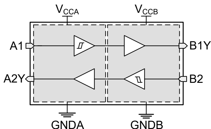
图 7-1. TXG4021 功能方框图
