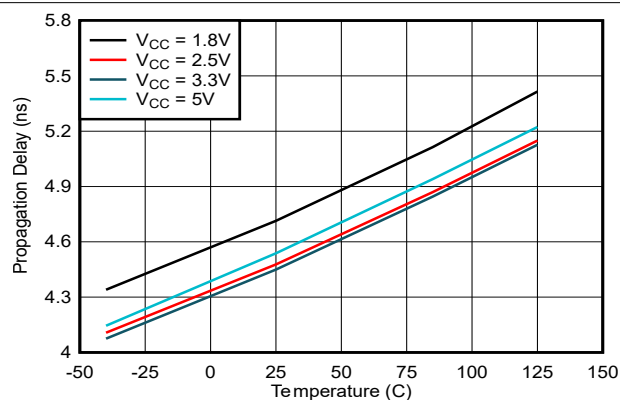
图 5-6. 传播延迟 T_{PLH} 与温度间的关系
