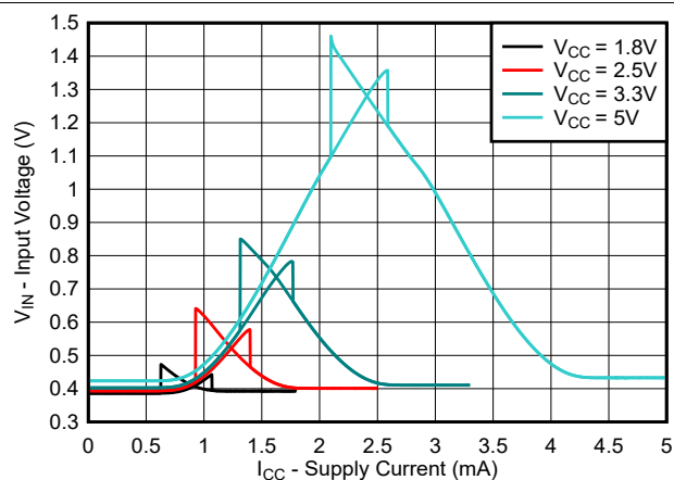
图 5-3. 电源电流 ( I_{CCA} ) 与输入电压 ( V_{IN} ) [TXG0x021] 间的关系
