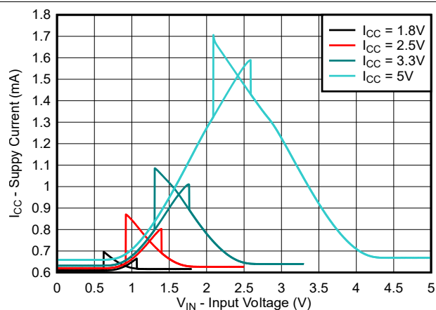
图 5-4. 电源电流 ( I_{CCB} ) 与输入电压 ( V_{IN} ) [TXG0x021] 间的关系
