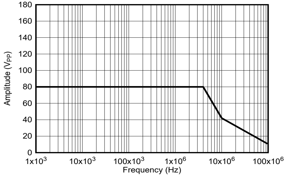
图 7-5. 交流噪声抑制图
