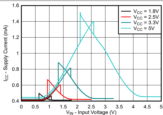
图 5-5. 电源电流 ( I_{CCA} ) 与输入电压 ( V_{IN} ) [TXGx020] 间的关系
