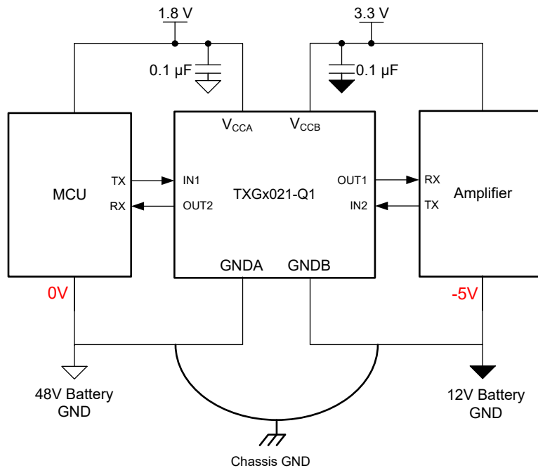
图 8-1. 汽车中的 TXG4021-Q1
