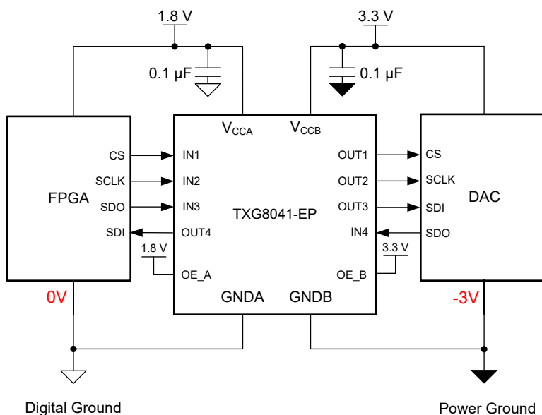
图 8-1. 航空电子设备中的 TXG8041-EP
