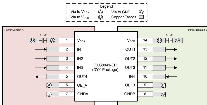
图 8-3. DYY 布局示例
