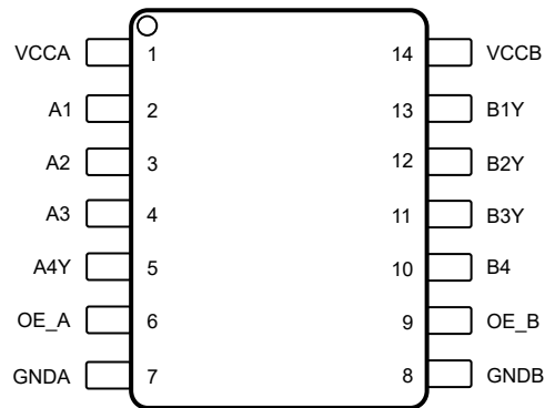
图 4-1. TXG8041-EP DYY 14 引脚 SOT 顶视图
