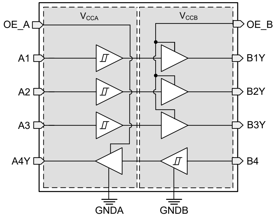
TXG8041-EP 功能方框图
