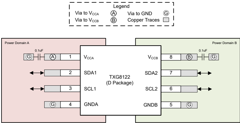
图 7-2. 布局示例 - TXG8122-Q1
