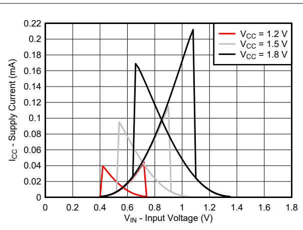
图 5-6. 典型 ( T_A=25^\circ\text{C} ) 电源电流 ( I_{CC} ) 与输入电压 ( V_{IN} ) 间的关系
