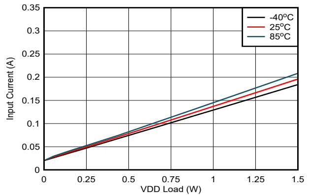
图 6-23. V_{VDD-VEE} 上输入电流与负载间的关系: V_{IN} = 15V , V_{VDD-VEE} = 22V , V_{COM-VEE} = 4V , V_{COM-VEE} 无负载
