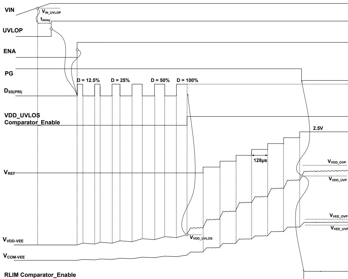
图 7-5. 输出电压软启动图
