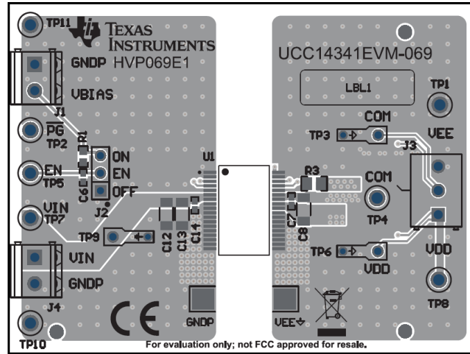
图 8-21. UCC14341-Q1EVM , PCB 顶层, 组装
