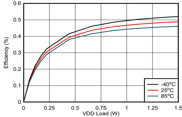
图 6-20. V_{VDD-VEE} 上效率与负载间的关系: V_{IN} = 16.5V , V_{VDD-VEE} = 22V , V_{COM-VEE} = 4V , V_{COM-VEE} 无负载
