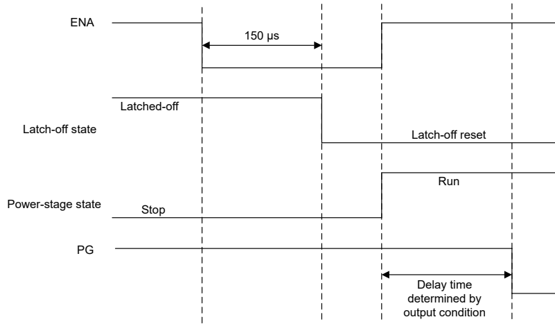
图 7-6. 使用 ENA 引脚的闭锁复位
