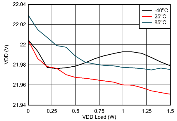
图 6-11. V_{VDD-VEE} 负载调节: V_{IN} = 15V , V_{VDD-VEE} = 22V , V_{COM-VEE} = 4V
