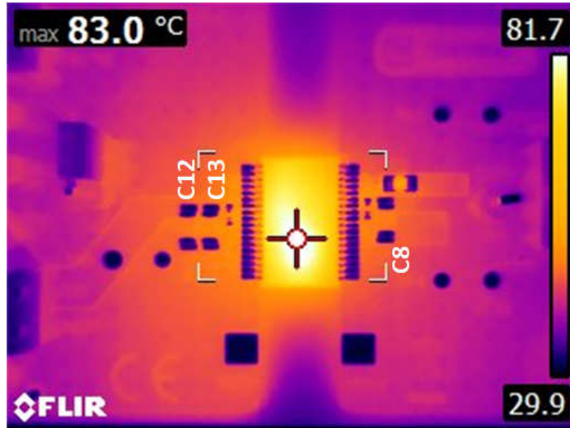
图 8-18. 热像图
