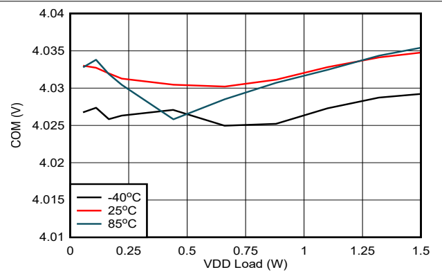
图 6-15. V_{COM-VEE} 负载调节: V_{IN} = 15V , V_{VDD-VEE} = 22V , V_{COM-VEE} = 4V
