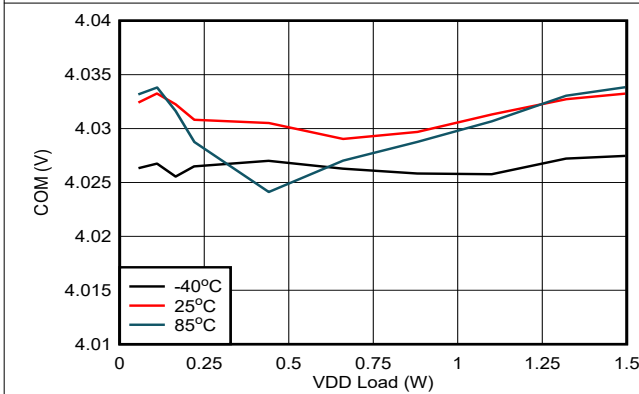
图 6-16. V_{COM-VEE} 负载调节: V_{IN} = 16.5V , V_{VDD-VEE} = 22V , V_{COM-VEE} = 4V
