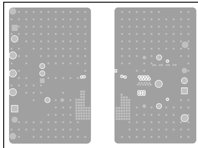
图 8-22. UCC14341-Q1EVM , 信号层 2 (与第 3 层相同)
