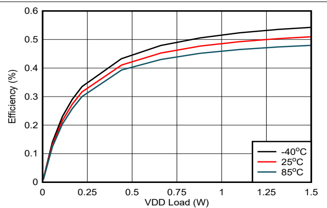
图 6-19. V_{VDD-VEE} 上效率与负载间的关系: V_{IN} = 15V , V_{VDD-VEE} = 22V , V_{COM-VEE} = 4V , V_{COM-VEE} 无负载
