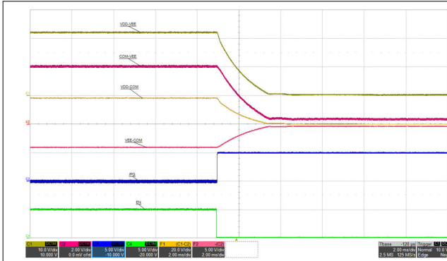
图 6-8. 关断: V_{IN} = 15V , V_{VDD-VEE} = 22V , V_{COM-VEE} = 4V , I_{VDD-VEE} = 68mA , V_{COM-VEE} 无负载。时间标度: 2ms/div。
