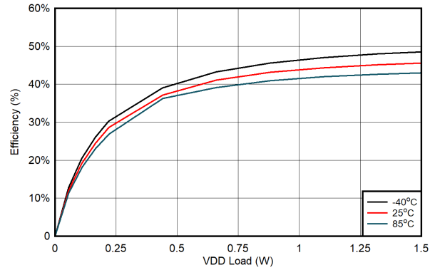
图 6-21. V_{VDD-VEE} 上效率与负载间的关系: V_{IN} = 18V , V_{VDD-VEE} = 22V , V_{COM-VEE} = 4V , V_{COM-VEE} 无负载
