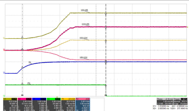
图 6-7. 启动: V_{\text{IN}} = 15\text{V} , V_{\text{DDD-VEE}} = 22\text{V} , V_{\text{COM-VEE}} = 4\text{V} , I_{\text{VDD-VEE}} = 68\text{mA} , V_{\text{COM-VEE}} 无负载。时间标度: 1ms/div。
