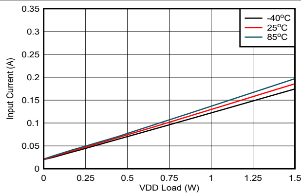
图 6-24. V_{VDD-VEE} 上输入电流与负载间的关系: V_{IN} = 16.5V , V_{VDD-VEE} = 22V , V_{COM-VEE} = 4V , V_{COM-VEE} 无负载
