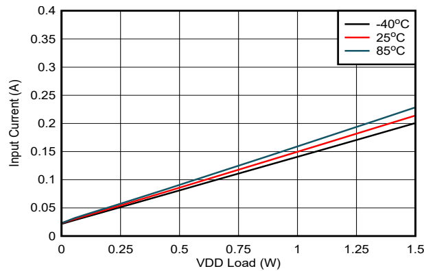
图 6-22. V_{VDD-VEE} 上输入电流与负载间的关系: V_{IN} = 13.5V , V_{VDD-VEE} = 22V , V_{COM-VEE} = 4V , V_{COM-VEE} 无负载
