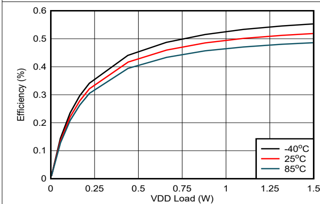
图 6-18. V_{VDD-VEE} 上效率与负载间的关系: V_{IN} = 13.5V , V_{VDD-VEE} = 22V , V_{COM-VEE} = 4V , V_{COM-VEE} 无负载
