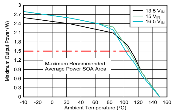
图 6-6. SOA 降额曲线: V_{\text{DDD-VEE}} = 22\text{V} , V_{\text{COM-VEE}} = 4\text{V} , T_{\text{shut}} = 150^{\circ}\text{C} , V_{\text{COM-VEE}} 无负载, 在屏蔽盒中测试。
