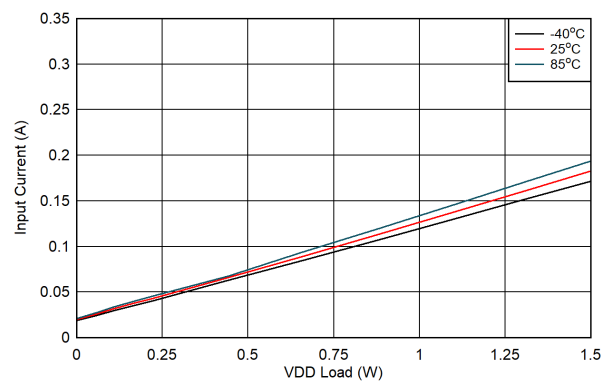
图 6-25. V_{VDD-VEE} 上输入电流与负载间的关系: V_{IN} = 18V , V_{VDD-VEE} = 22V , V_{COM-VEE} = 4V , V_{COM-VEE} 无负载
