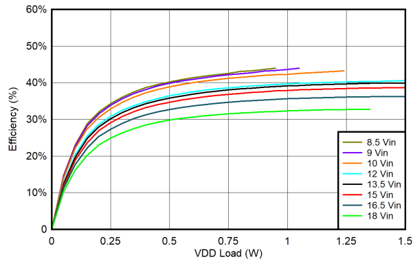
图 6-32. UCC14341B-Q1 V_{VDD-VEE} 上效率与负载间的关系: T_{AMBIENT} = 85^{\circ}C , V_{VDD-VEE} = 15V , V_{COM-VEE} = 4V , V_{COM-VEE} 无负载
