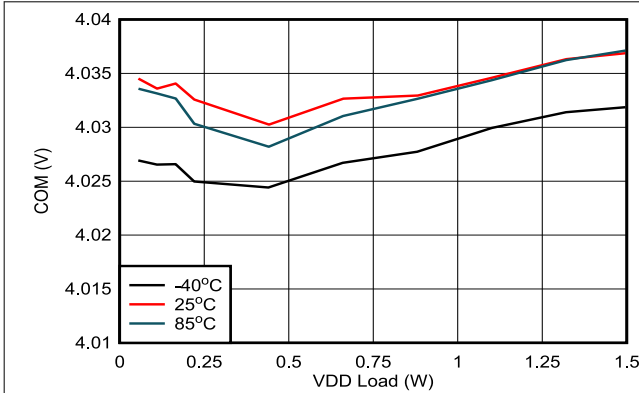
图 6-14. V_{COM-VEE} 负载调节: V_{IN} = 13.5V , V_{VDD-VEE} = 22V , V_{COM-VEE} = 4V
