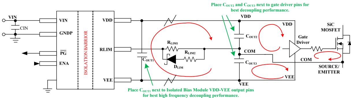
图 8-3. 具有 C_{out1} 、 C_{out2} 和 C_{out3} 的双路输出原理图
