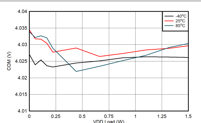
图 6-17. V_{COM-VEE} 负载调节: V_{IN} = 18V , V_{VDD-VEE} = 22V , V_{COM-VEE} = 4V
