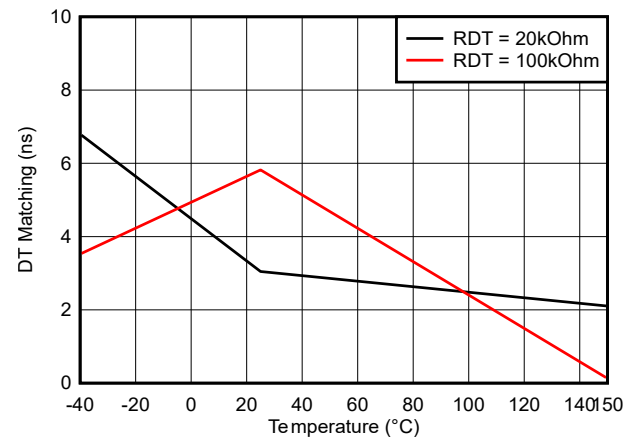
图 5-27. 死区时间匹配与温度之间的关系 (R DT = 20kΩ 和 100kΩ)
