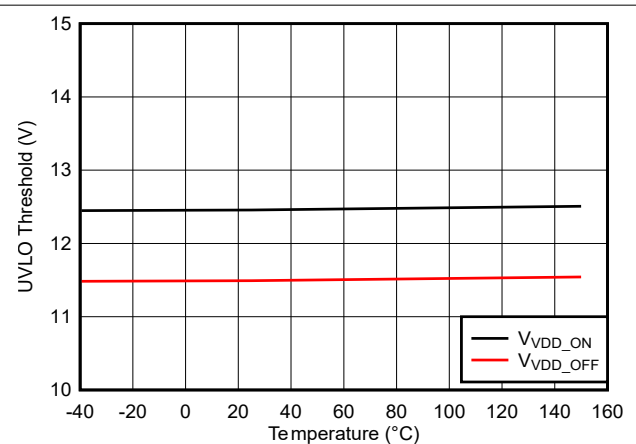
图 5-21. VDD 12V UVLO 阈值与温度之间的关系
