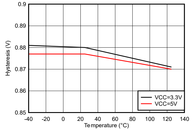
图 5-23. IN/DIS 迟滞与温度之间的关系
