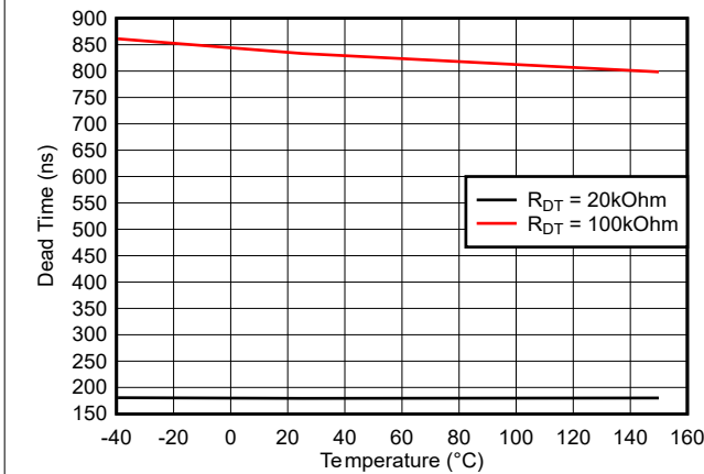
图 5-26. 死区时间与温度之间的关系 (R DT = 20kΩ 和 100kΩ)
