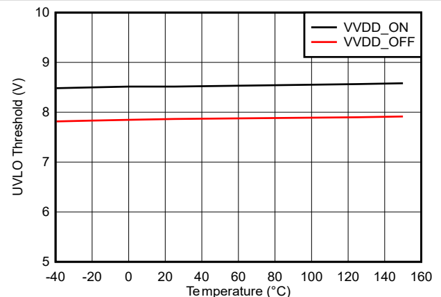
图 5-19. VDD 8V UVLO 阈值与温度之间的关系
