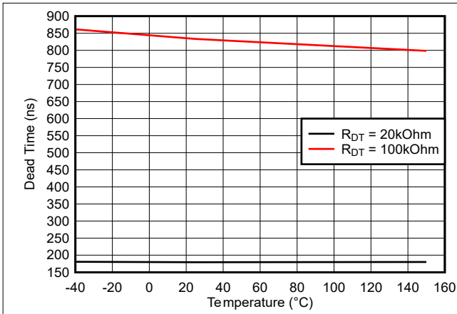
图 5-21. 死区时间与温度之间的关系 ( R DT = 20kΩ 和 100kΩ )
