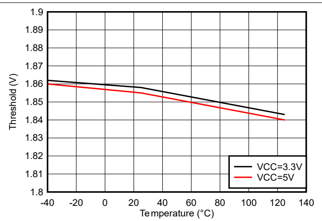
图 5-20. IN/EN 高阈值
