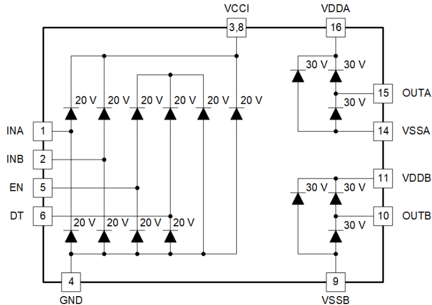
图 8-3. ESD 结构
