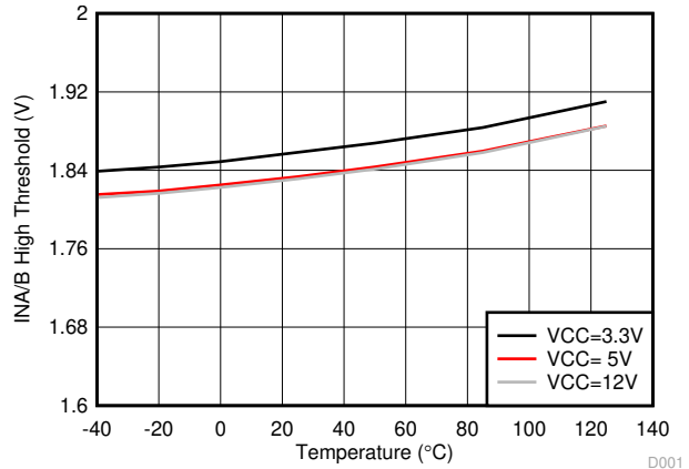
图 6-23. INA/B 高阈值
