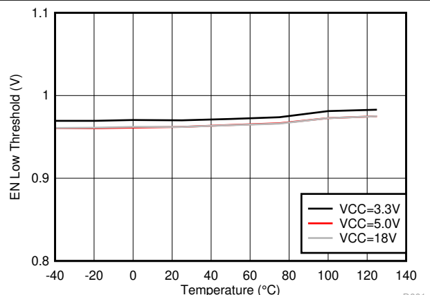
图 6-25. EN 低阈值
