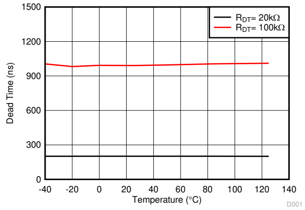
图 6-27. 死区时间与温度之间的关系 (R DT = 20kΩ / 100kΩ)
