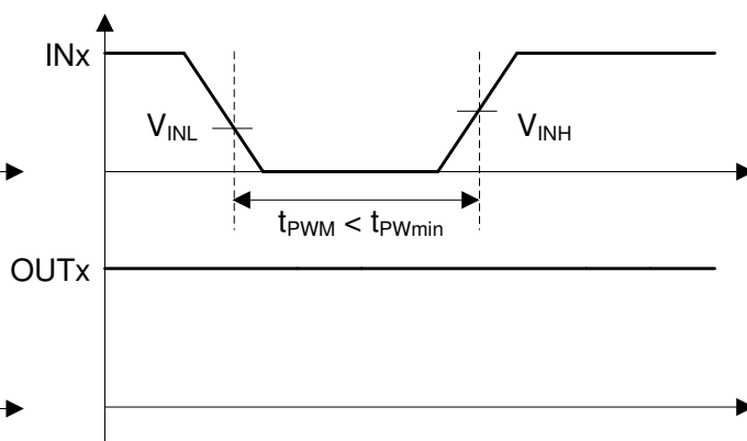
图 7-2. 抗尖峰脉冲滤波器 - 关断
