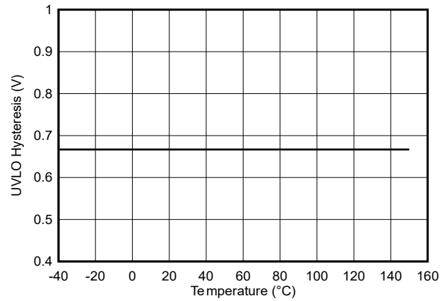
图 6-13. 8V VDD UVLO 阈值迟滞电压
