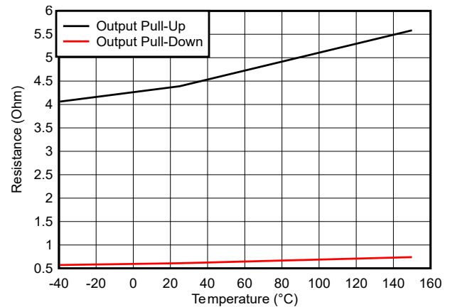
图 6-15. OUT 上拉和下拉电阻
