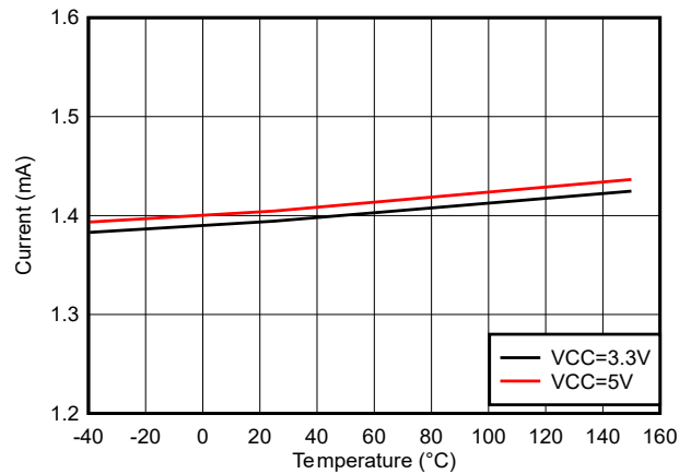
图 5-11. I_{VCCI} 静态电源电流与温度之间的关系 (无负载, 低电平输入, 无开关)
