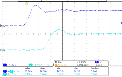
图 7-5. HO 上升时间和 HI 至 HO 导通传播延迟
