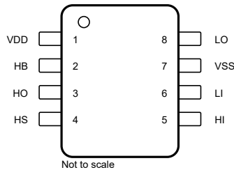
图 4-2. D 封装 8 引脚 SOIC 底视图
