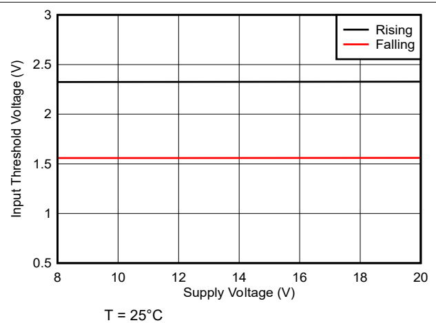
图 5-5. 输入阈值与电源电压间的关系
