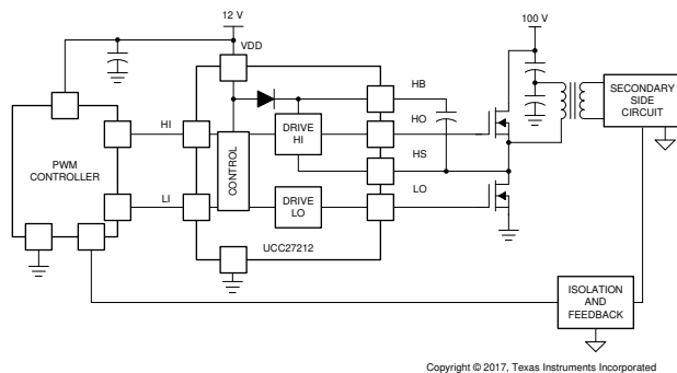
典型应用图
