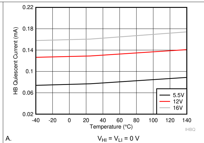
图 6-2. HB Quiescent Current
