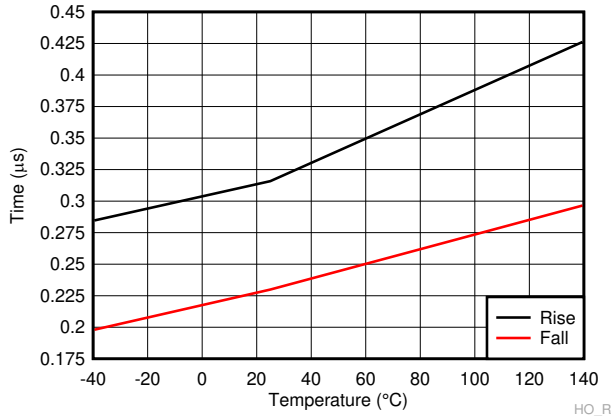
图 6-27. HO Rise & Fall Time
