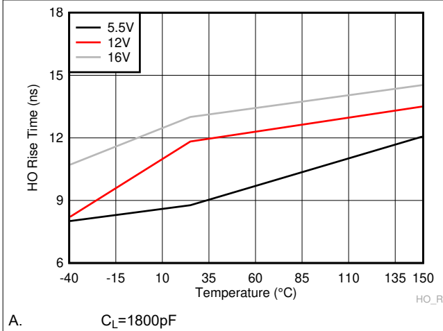
图 6-19. HO Rise Time
