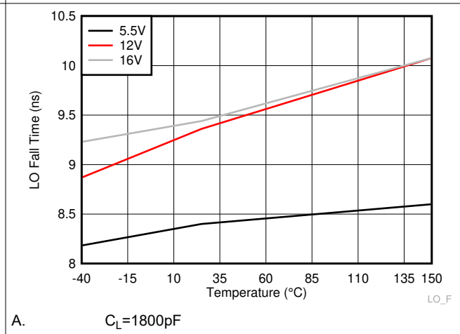
图 6-18. LO Fall Time
