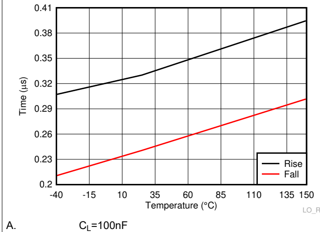
图 6-21. LO Rise andamp; Fall Time
