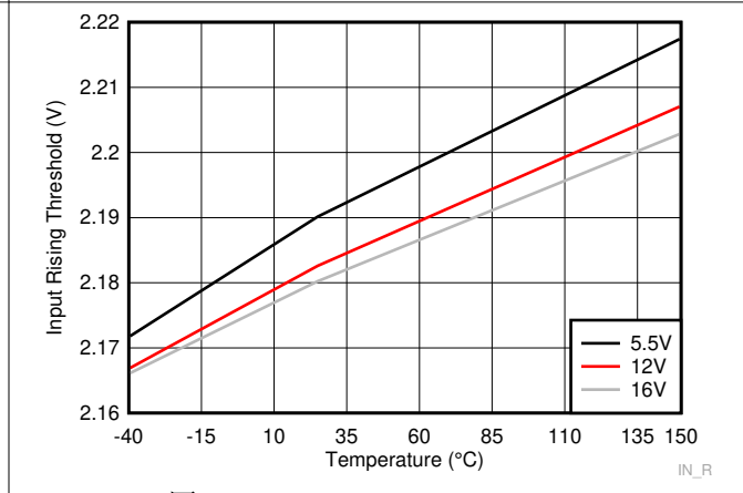
图 6-6. Input Rising Threshold
