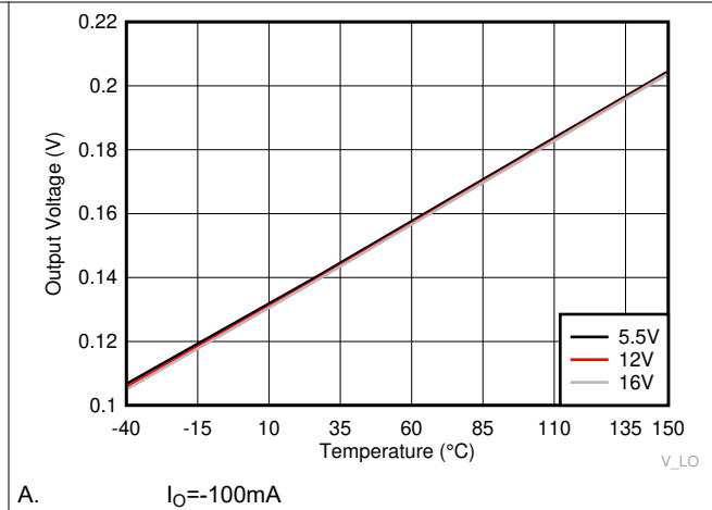
图 6-14. LO High Output Voltage ( V_{LOH} )
