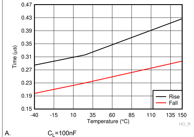
图 6-22. HO Rise andamp; Fall Time
