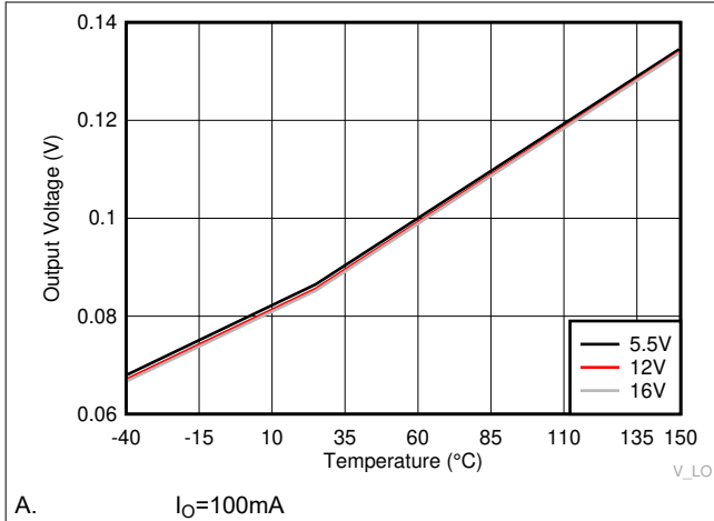
图 6-13. LO Low Output Voltage ( V_{LOL} )
