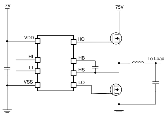
简化版应用示意图
