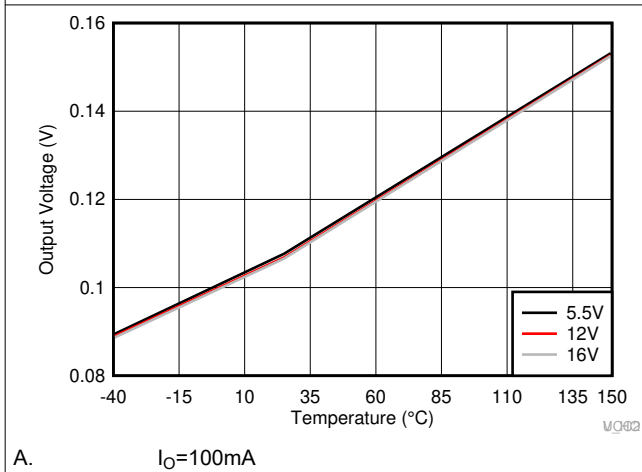
图 6-15. HO Low Output Voltage ( V_{HOL} )
