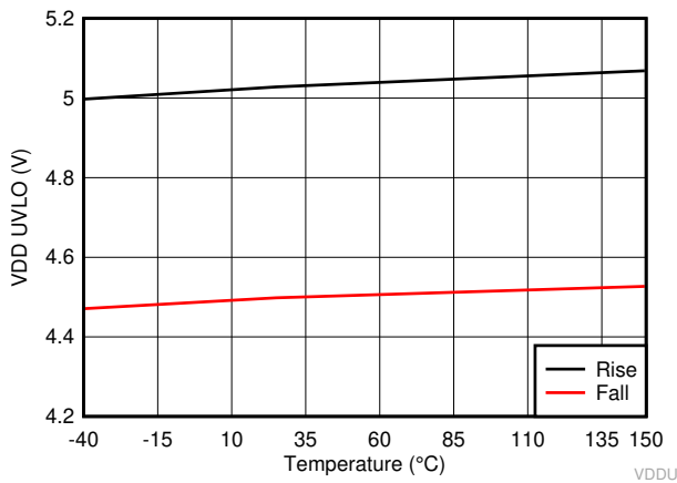
图 6-9. VDD UVLO Threshold
