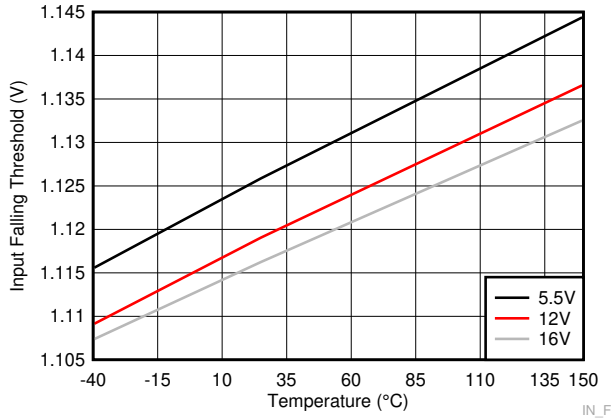
图 6-7. Input Falling Threshold
