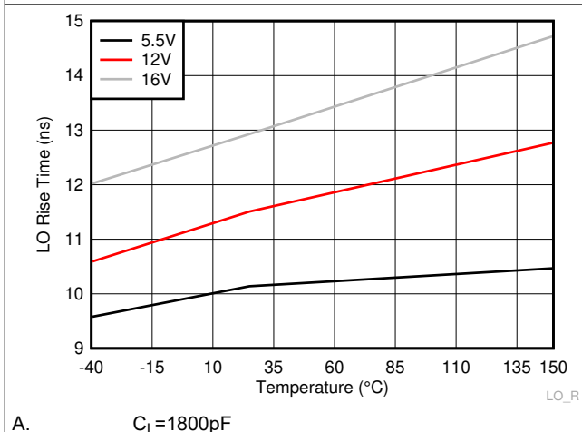
图 6-17. LO Rise Time
