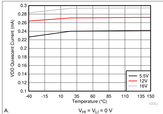
图 6-1. VDD Quiescent Current
