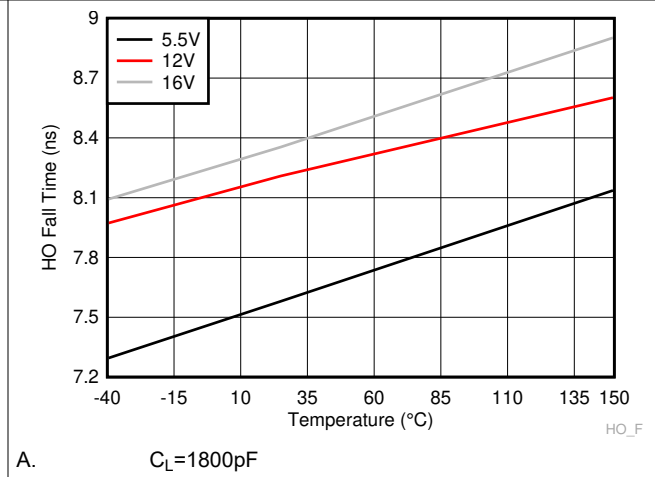
图 6-20. HO Fall Time
