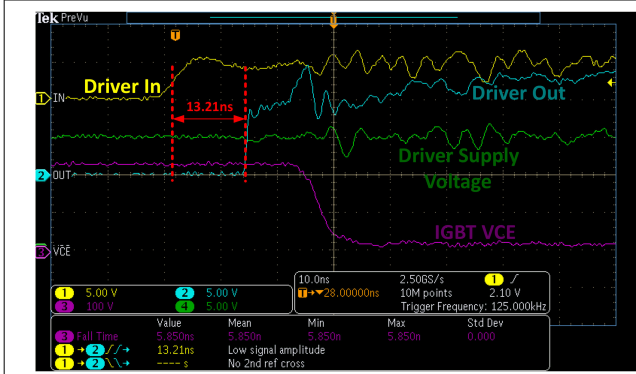
图 7-4. 导通传播延迟波形
