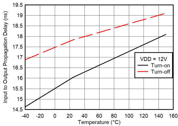
图 5-19. 输入传播延迟与温度间的关系
