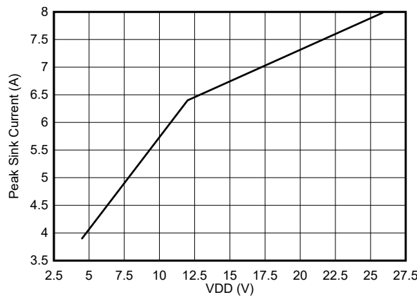
图 5-25. 峰值灌电流与 VDD 间的关系
