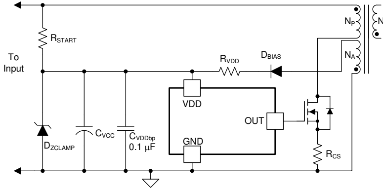
图 7-1. VDD 保护
