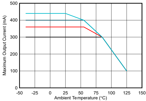
图 6-3. 最大输出电流与环境温度间的关系 : VCC = 5.0V, C OUT2 = 22 μF
