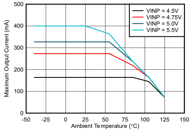
图 6-4. 最大输出电流与环境温度间的关系 : VCC = 5.5V, C OUT2 = 22 μF
