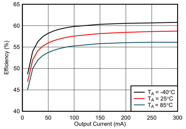
图 6-6. 效率与负载电流 (I VCC ) 间的关系 : VCC = 5.0V, VINP = 5.0V, C OUT2 = 22 μF
