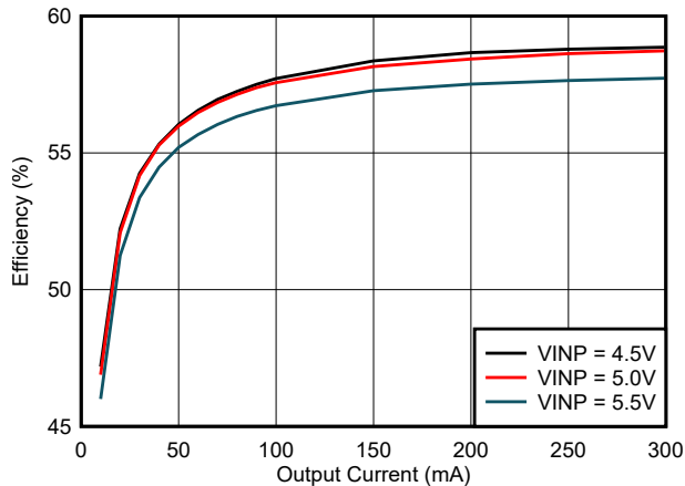
图 6-5. 效率与负载电流 (I VCC ) 间的关系 : VCC = 5.0V, T A = 25°C, C OUT2 = 22 μF
