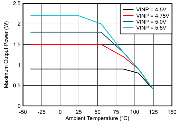
图 6-2. 最大输出功率与环境温度间的关系 : VCC = 5.5V, C OUT2 = 22 μF
