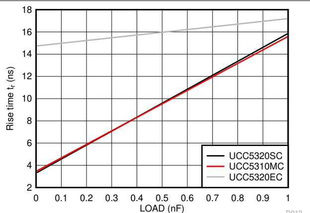
图 6-36. Rise Time vs Load Capacitance
