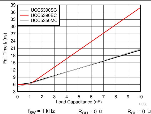
图 6-40. Fall Time vs Load Capacitance
