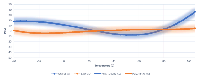
그림 4. BAW 오실레이터와 쿼츠의 온도 안정성 비교
