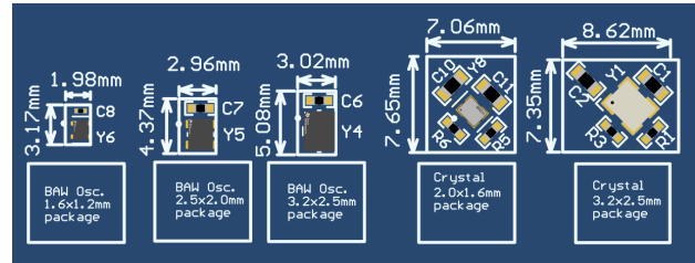
그림 2. BAW 오실레이션과 크리스탈의 PCB 풋프린트 비교
