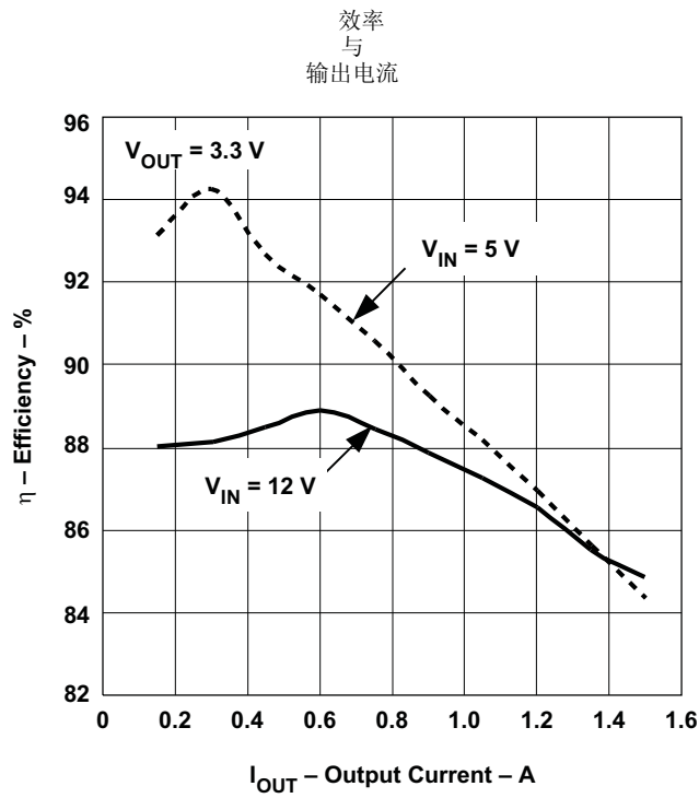
图 9. TPS62111 效率性能
