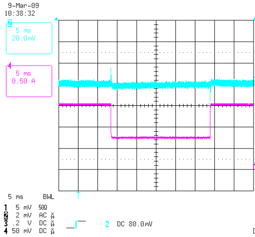
图 7. 750mA 与 1.5A 之间的负载步进瞬变, V_{IN} = 12V
