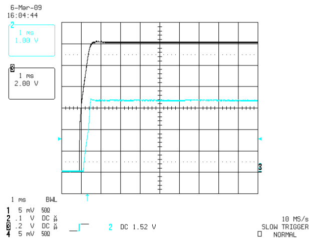
图 4. 启动 V_{IN} = 12V , 无负载
