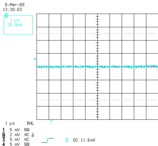
图 5. 输出纹波电压, V_{IN} = 5V
