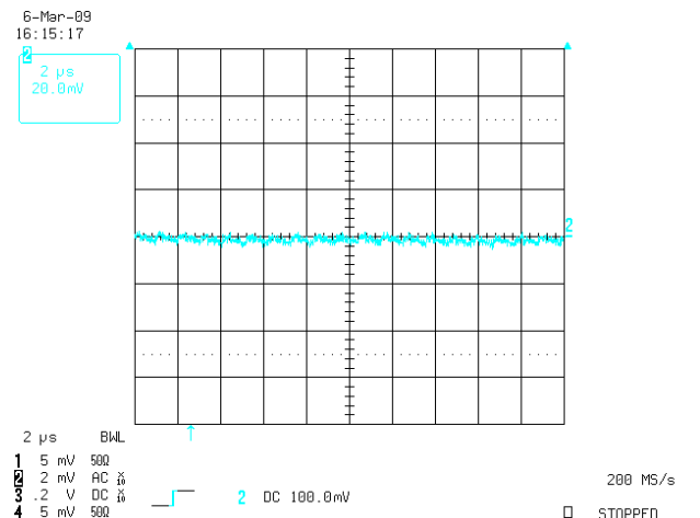
图 6. 输出纹波电压, V_{IN} = 12V
