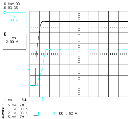
图 3. 启动 V_{IN} = 12V , I_{LOAD} = 1.5A
