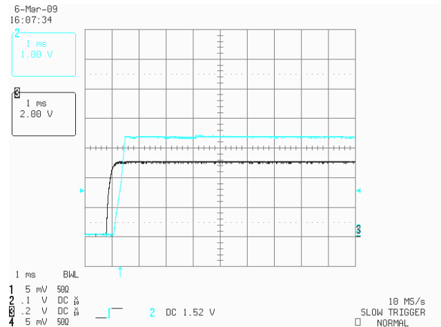
图 2. 启动 V_{IN} = 5V , 无负载
