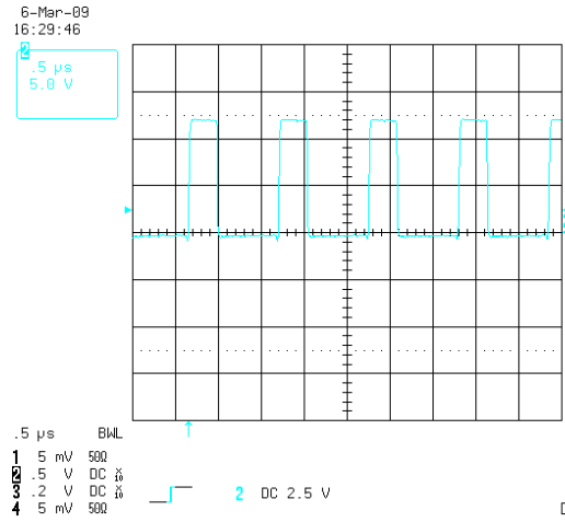
图 8. 开关节点波形, V_{IN} = 12V
