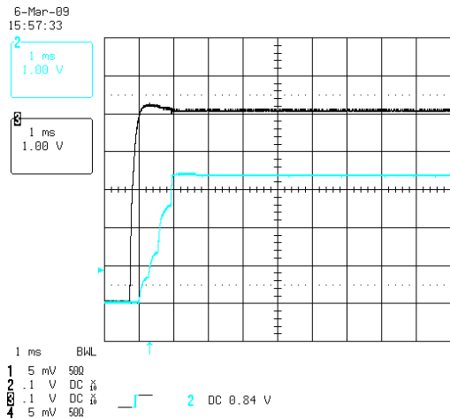
图 1. 启动 V_{IN} = 5V , I_{LOAD} = 1.5A
