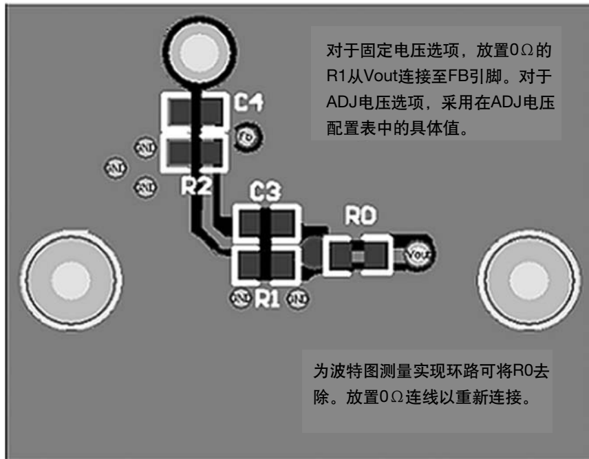
图6. 底层布局(SOT 23-5)
