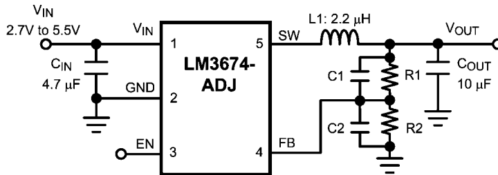
图2. 典型的应用电路
