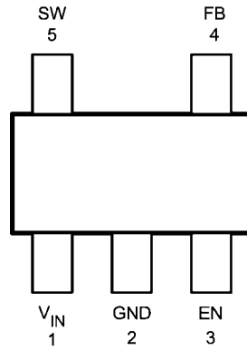
图3. SOT23-5 封装, 顶视图
