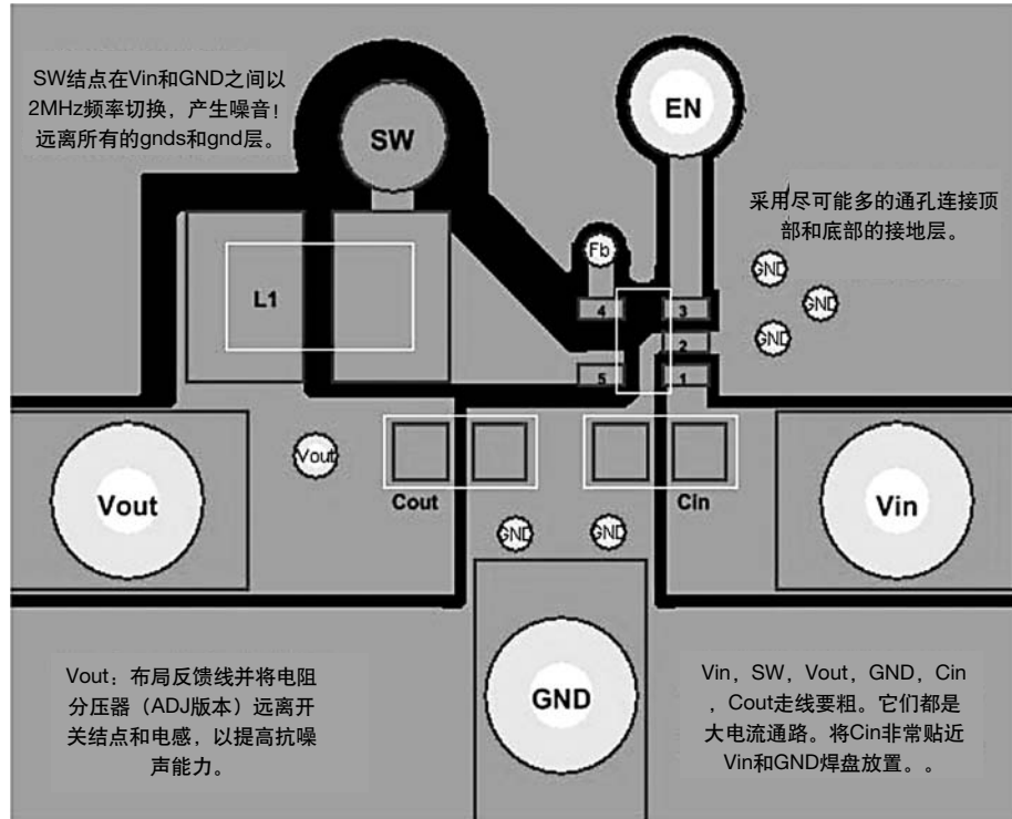
图4. 顶层布局 (SOT 23-5)
