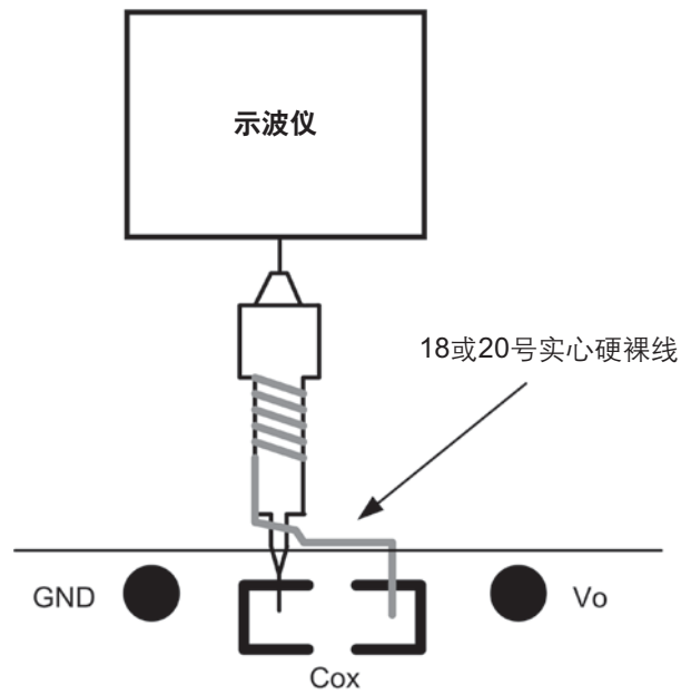
图5. 输出电压纹波测量的设置
